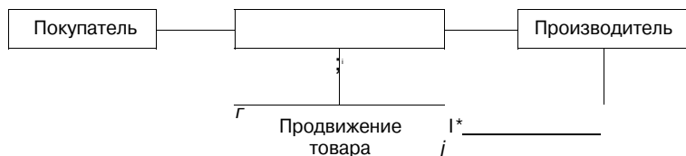
Рис. 9.3. Проталкивание товара
